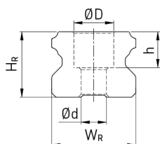
Mål på profilskinne EGR_U
